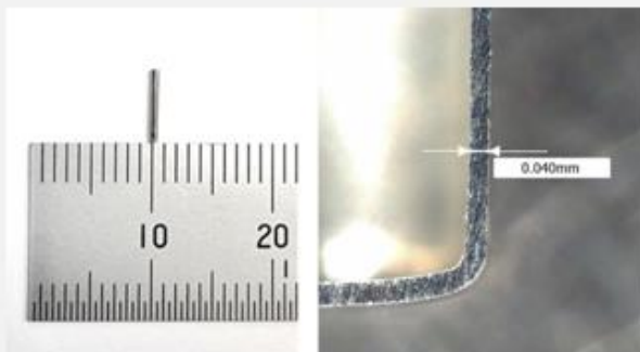
SUS316L 極細極薄絞り
